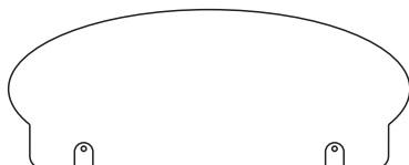
Formfräsung Ovaleck 2er DWT 960 x 380 Fräsform
