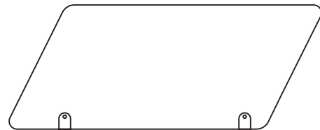
Formfräsung Diagonaleck 4er DWT Abmessung 1180 x 470 mm
