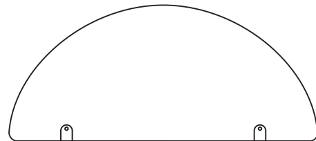
Formfräsung Rundeck 4er DWT Abmessung 1180 x 520 mm
