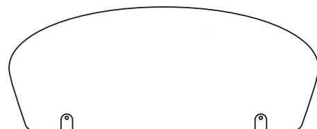
Formfräsung Ovalrundeck 4er DWT Abmessung 1180 x 470 mm
