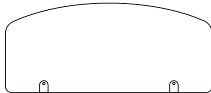
Formfräsung Bogeneck 4erDWT Abmessung 1080 x 470 mm
