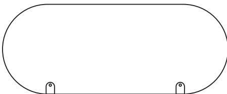
Formfräsung Rundradiuseck 4er DWT Abmessung 1180 x 470 mm
