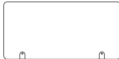
Formfräsung Radieneck Taxi 4er DWT Abmessung 1000 x 490 mm
