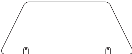
Formfräsung Trapezeck 4er DWT Abmessung 1180 x 470 mm
