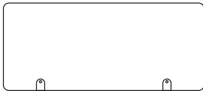
Formfräsung Radieneck 4er DWT Abmessung 1080 x 470 mm
